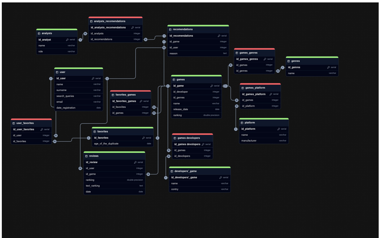
Рисунок 1 - Физическая схема данных
